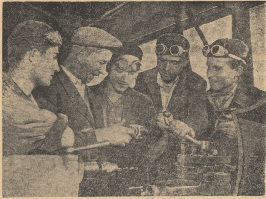
Maistrul strungar Ion Drăgulin de la școala Băleni ralonul Tg. Jiu regiunea Craiova explică tinerilor Părin Constantin, Gh. Toma, Ion Colot și Alion Vasile felul cum trebuie lucrat un ventil de încălzire pentru capetele de erupție.
