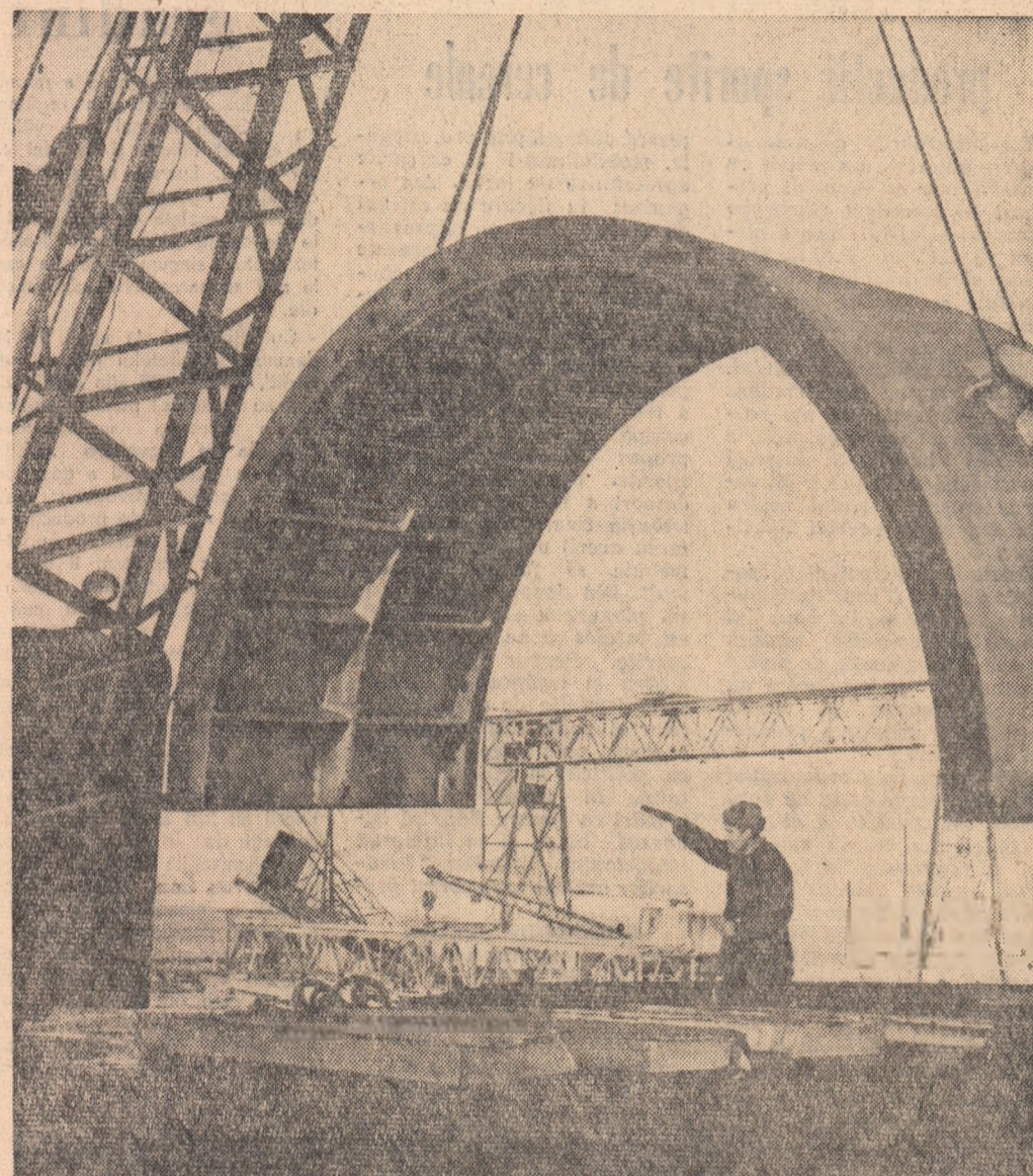
Descărcarea unei părți a urzei turbine de aburi care va deservi termocentrala electrică de la Cernetsk (U.R.S.S.), termocentrală în curs de construcție.
