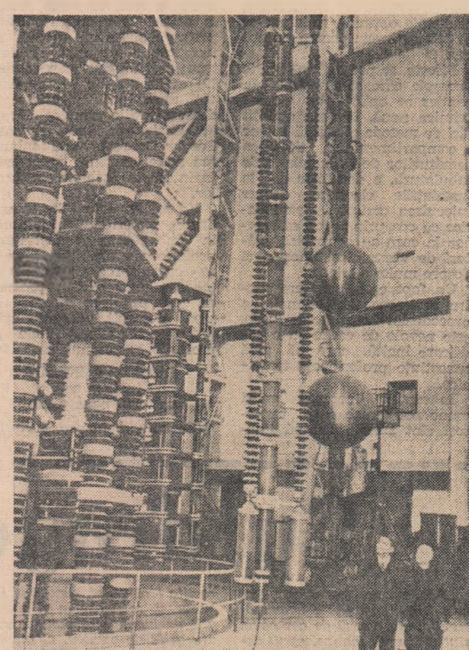
În hala Institutului unional de electrotehnică „V. I. Lenin” pentru încercarea transformatorilor și a altor aparate electrice de înaltă tensiune. Foto: TASS-MOSCOVA
