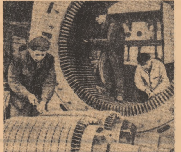
R. P. D. COREANĂ. — Muncitorii ai Uzinei electrotehnice din Than executînd lucrări de montaj
