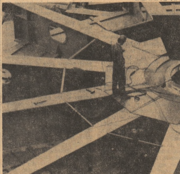
Asamblarea rotorului turbinei 6 de la Porțile de Fier
