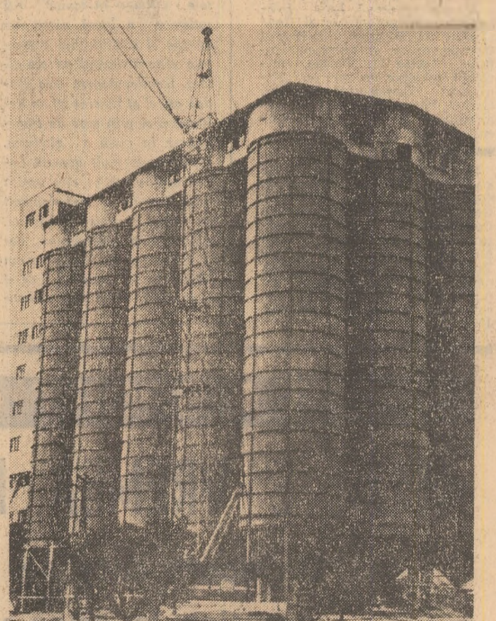
R.S. CEHOSLOVACA. — Specialiștii din Pardubice au pus la punct o nouă tehnologie de construcție a silozurilor. În fotografie, primul dintre acestea înălțat cu ajutorul noii tehnologii.
