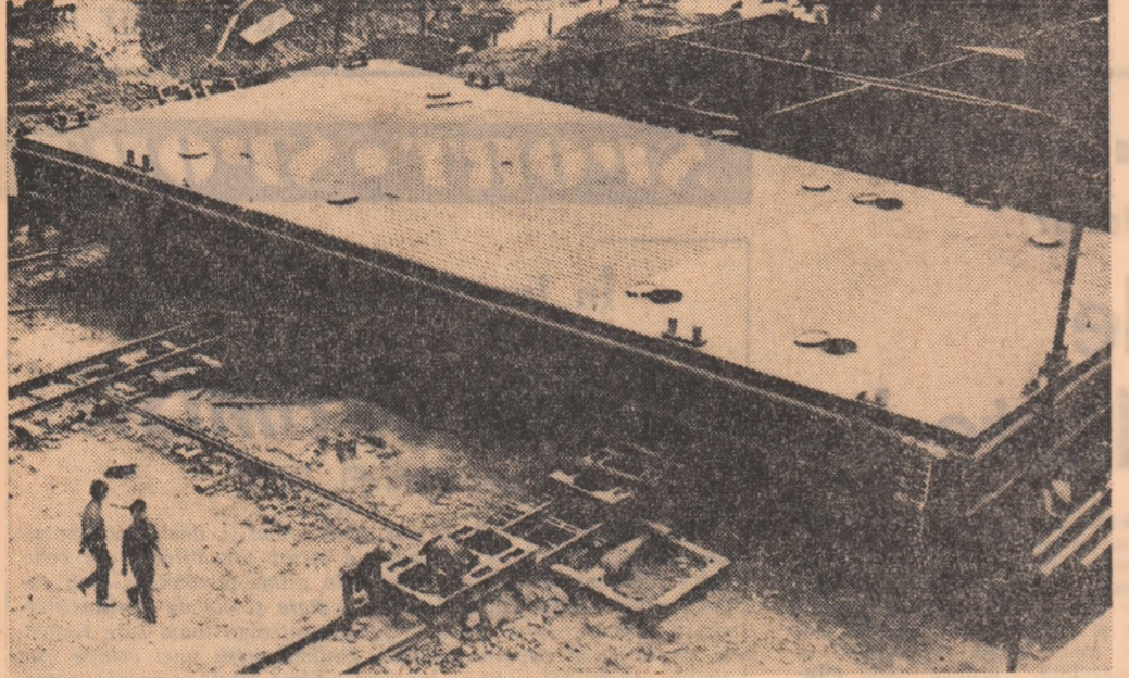
R.D. VIETNAM: Realizarea la întreprinderea constructoare de mașini An Bien a unei dane plutoare de acostare.
