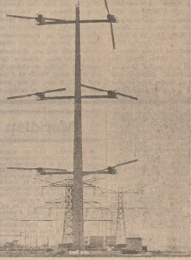
În întreaga lume se depun eforturi în vederea aplicării unor alternative energetice, care să conducă atât la economia de energie, cit și la reducerea drastică a poluării atmosferice. În imagine: sistem multiplu eolian instalat în Olanda la o înălțime de peste 50 de metri, care, cu cele 6 brațe ale sale, are o capacitate de circa 450 kW
