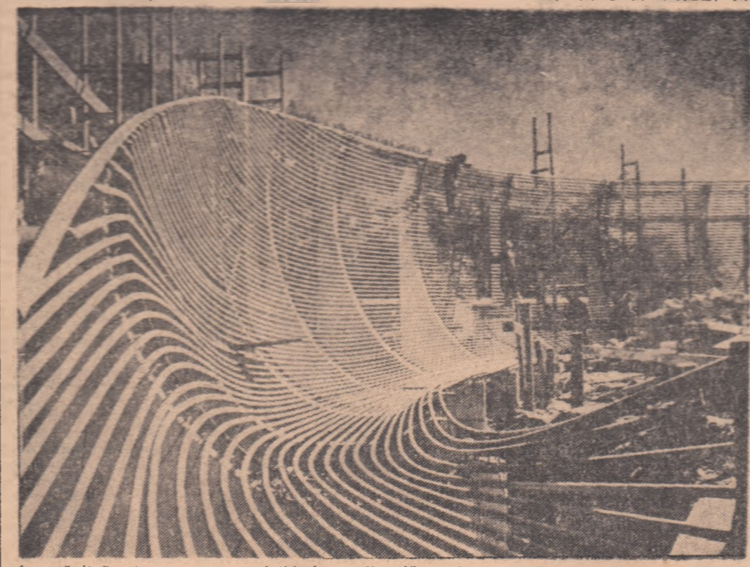
Această fină rețea pe care o vedeți în fotografia alăturată constituie infrastructura pîrtiei pe care se vor desfășura la 1 și 2 februarie a.c. campionatele mondiale de săniute. Pîrtia se construiește la Königssee în apropierea stațiunii Berchtesgaden (R.F.G.) și este prima din lume realizată cu gheață artificială. Pentru cei 1114 metri ai acestei pîrtii s-au consumat 55 km de feață pentru răcire
