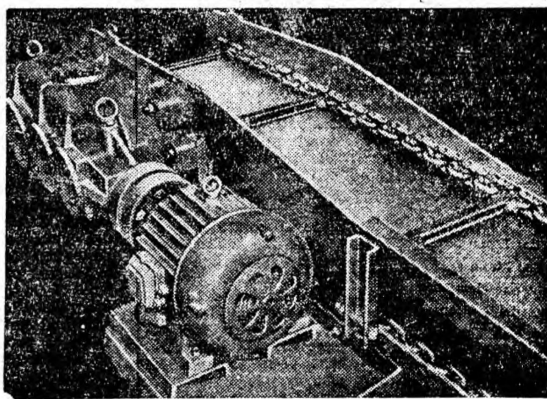
În frontalul de pe stratul 15 panoul 1 la sectorul IV B Lupeni, funcționează de mai bine de o lună un utilaj modern de mare capacitate: transportorul PZP-45 adus în Valea Jiului din R.P. Polonă. Transportorul acesta (vezi clișeu) este blindat, permițînd astfel havarea de pe el. Cu ajutorul său brigada condusă de Panțiru Ioan obține un randament mediu de peste 4 tone cărbune pe post și extrage o fișie de cărbune pe zi.
