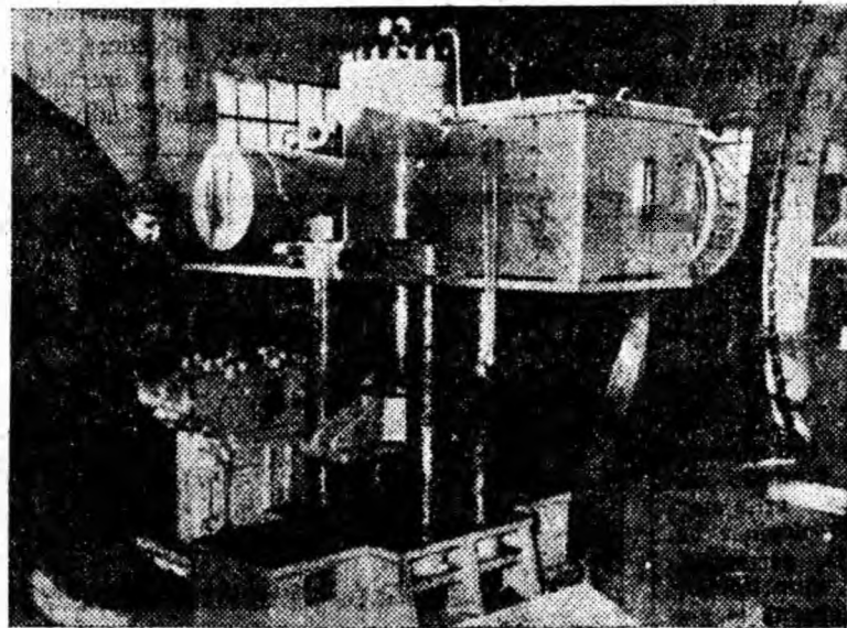
La atelierul mecanic al minei Lupeni a fost pusă de curind în funcțiune o presă hidraulică de 100 tone cu ajutorul căreia pot fi recondiționați stîlpi de abataj curbați din cauza presiunii. ÎN CLIȘEU: Noua presă modernă, dotată cu dispozitive de comandă de la distanță.
