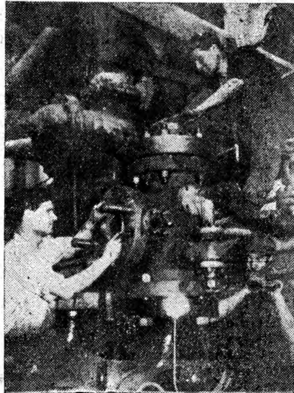
La termocentrala Paroșeni se montează o nouă electropompă. IN CLIȘEU: Aspect din timpul montării.
