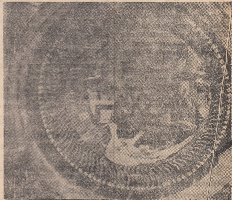
La U. E. Vulcan (secția A.C.R.E.V.) un nou stator de 300 kilowați va fi reparat înainte de termen. ÎN CLIȘEU: Bobinatorii Pietraru Constantin și Cîndea Maria, fruntași în întrecerea socialistă, lucrînd la stator.
