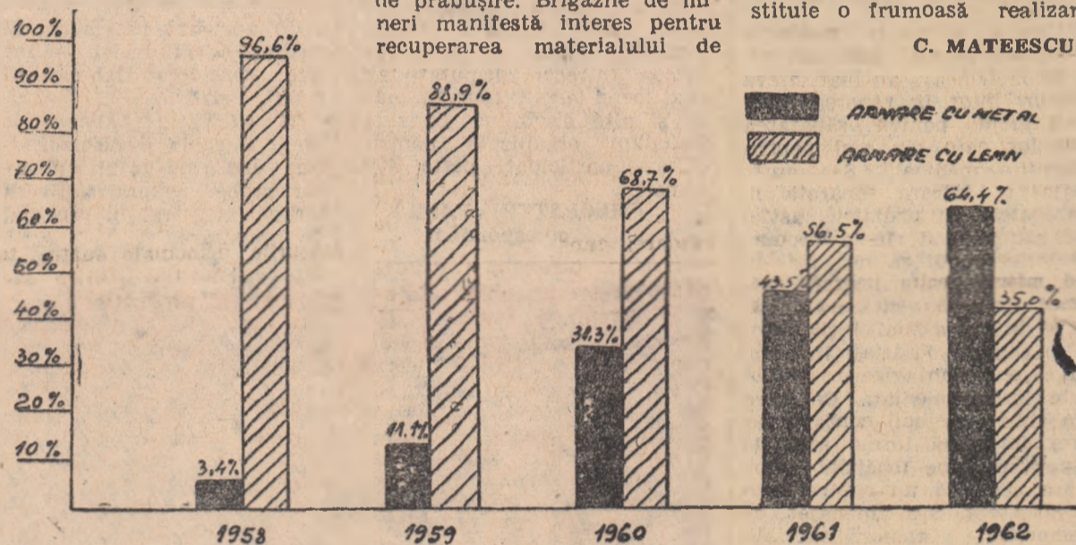
Graficul înfățișează dinamica extinderii armării metalice în abatajele minei Lupeni și a reducerii consumului de lemn.
