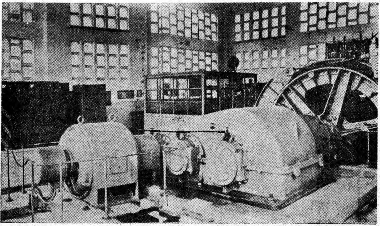
CASA MAȘINII DE EXTRAȚIE DE LA PUȚUL AUXILIAR NR. 3 DÎLJA.
