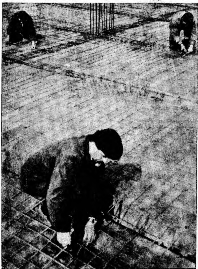
Vasta armătură a planșului de la construcția noii clădiri a băii-lămpăriei minei Uricani, este „tesută” cu pricepere de fierar-betonistiți din brigada lui Firjöl Gheorghe.
