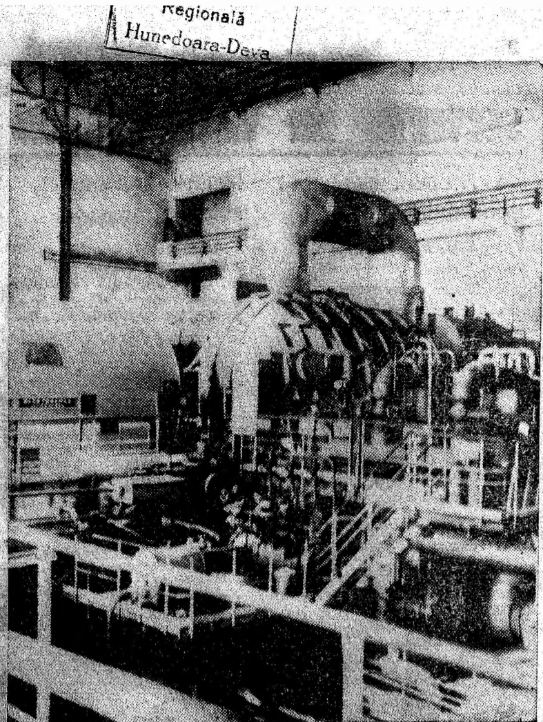
Turbogeneratorul nr. 4 de la I.E.C. Paroșeni. Acesta poate „pompa” în fiecare oră 150 MW energie electrică în sistemul energetic.
