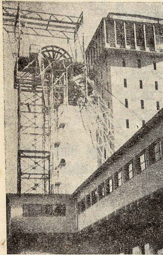
LONEA II: Complexul de extracție: puțul vechi metalic și alături, puțul nou cu schip, ridicat din beton.
