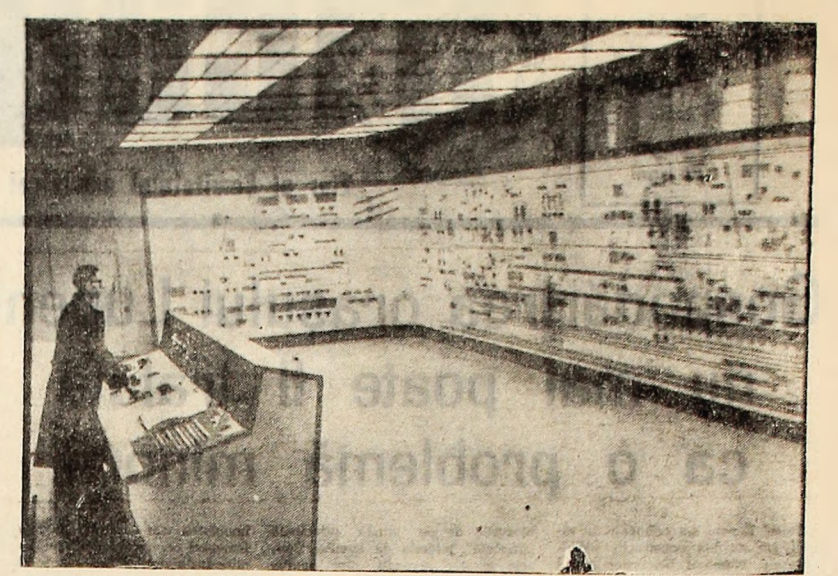
PREPARAȚIA COROȘTII: Aspect din sala de comană centralizată a instalațiilor de preparare a carbunilor.
