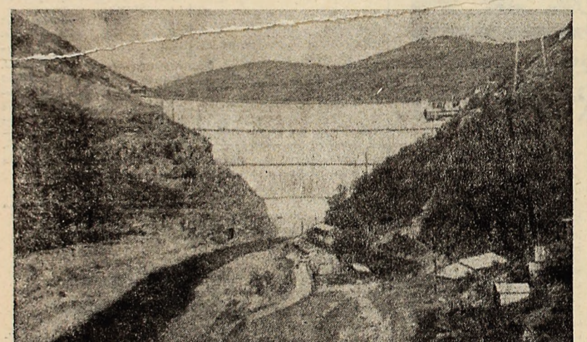
R.S.J. IUGOSLAVIA: Partea a sistemului hidro-energetic Trebisnjica, hidrocentrala Granciarevo este una din centralele de mare putere ale sistemului, urmînd să producă 2.000 KWH. IN CIUȘEU: Vederea a barajului Granciarevo.
