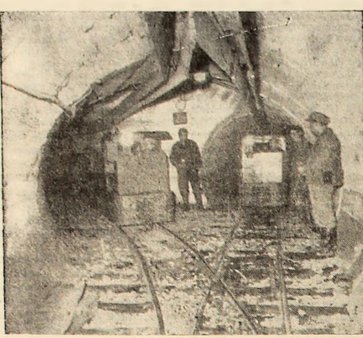
Galeriile de garare a vagonetelor de la pătul sud — Aninoasa.
