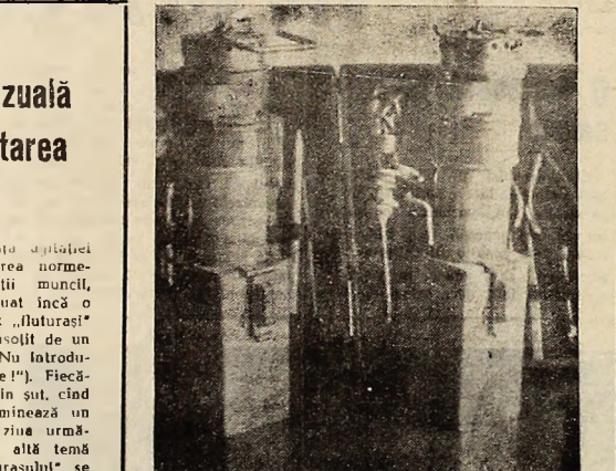
Metanometre pentru măsurarea concentrației de gaz metan în atmosfera locurilor de muncă din subteran.
