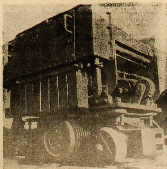
Inelele metalice și căptușeala suplă din plasă de sîrmă conferă spațiu încăpător și trîncinie suitorului săpat cu foreza Hausssher. Aplicarea noului sistem de săpare, pe lângă faptul că scurtează timpul de execuție la mai mult de jumătate, permite reducerea substanțială a materialului lemnos.
