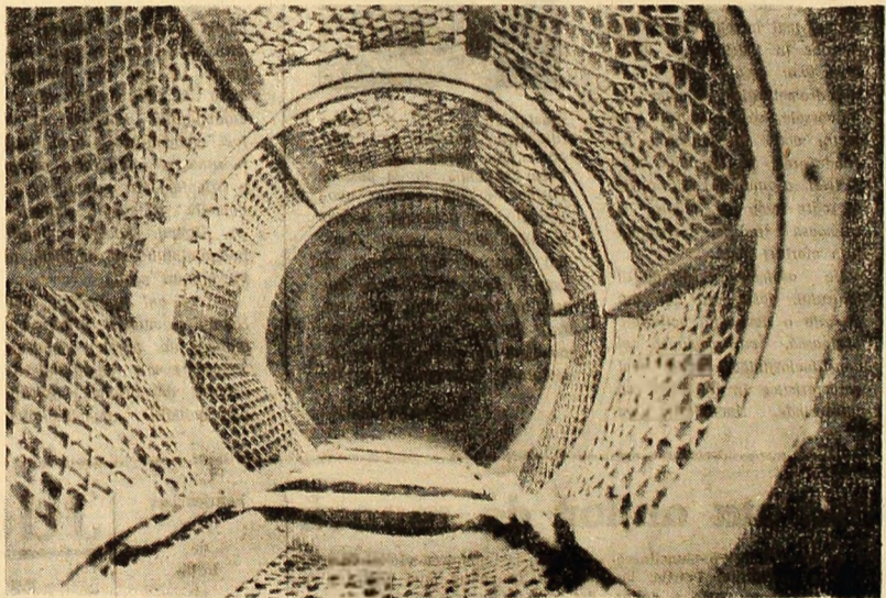
Inelele metalice și căptușeala suplă din plasă de sîrmă conferă spațiu încăpător și trîncinie suitorului săpat cu foreza Hausssher. Aplicarea noului sistem de săpare, pe lângă faptul că scurtează timpul de execuție la mai mult de jumătate, permite reducerea substanțială a materialului lemnos.
