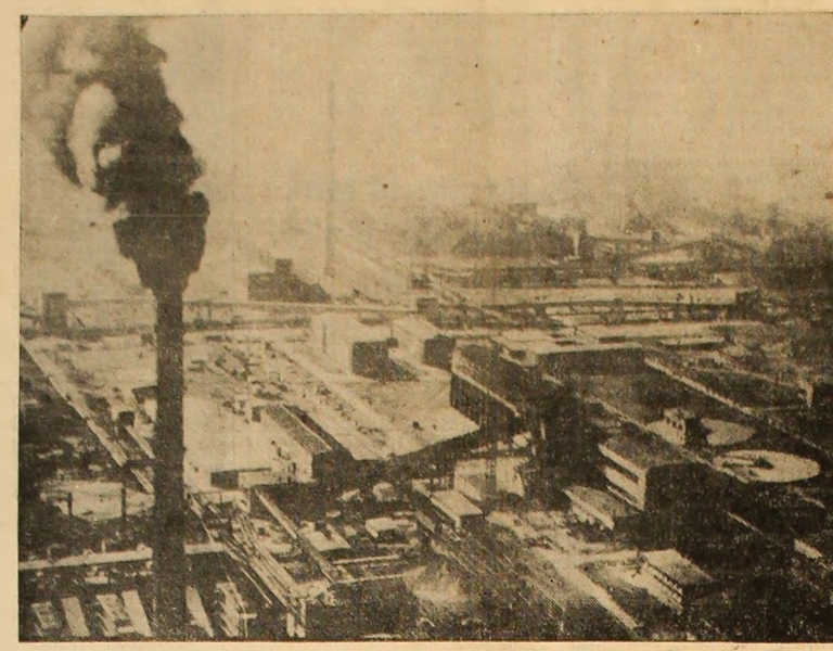
R. P. BULGARIA: Vedere aeriană a instalațiilor metalurgice Kremikovski, situate în apropiere de Sofia.
