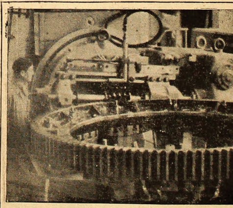
Aspect din hala de mecanică grea a U.U.M.P. Foto: A. DULA
