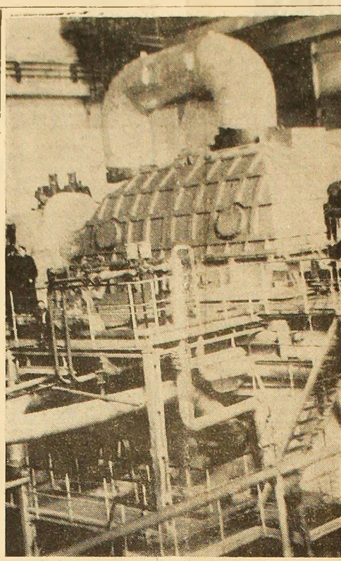
Termocentrala Paroseni. Sala turbogeneratoarelor
