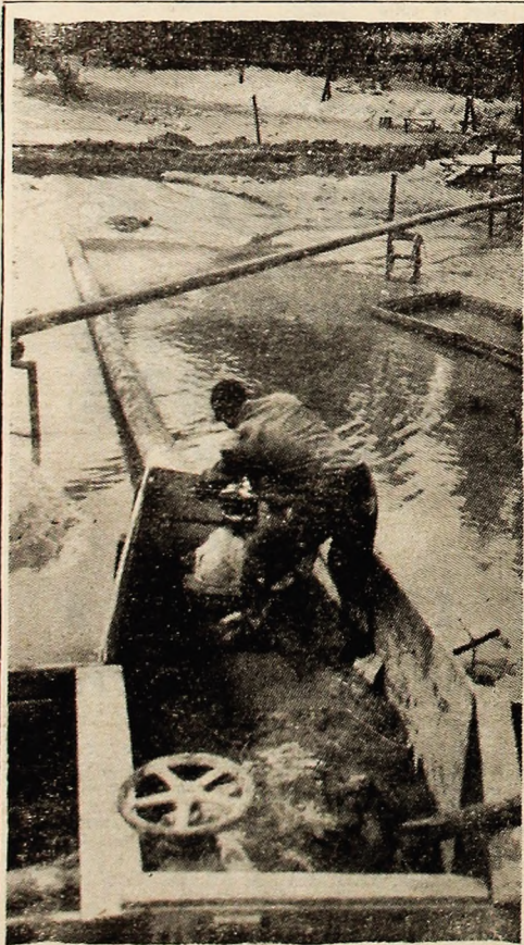
Exploatarea minieră Deva. Se lucrează la degajarea stațiilor de pompe (desfundarea conductelor) la iazul de decantare a sterilului.
