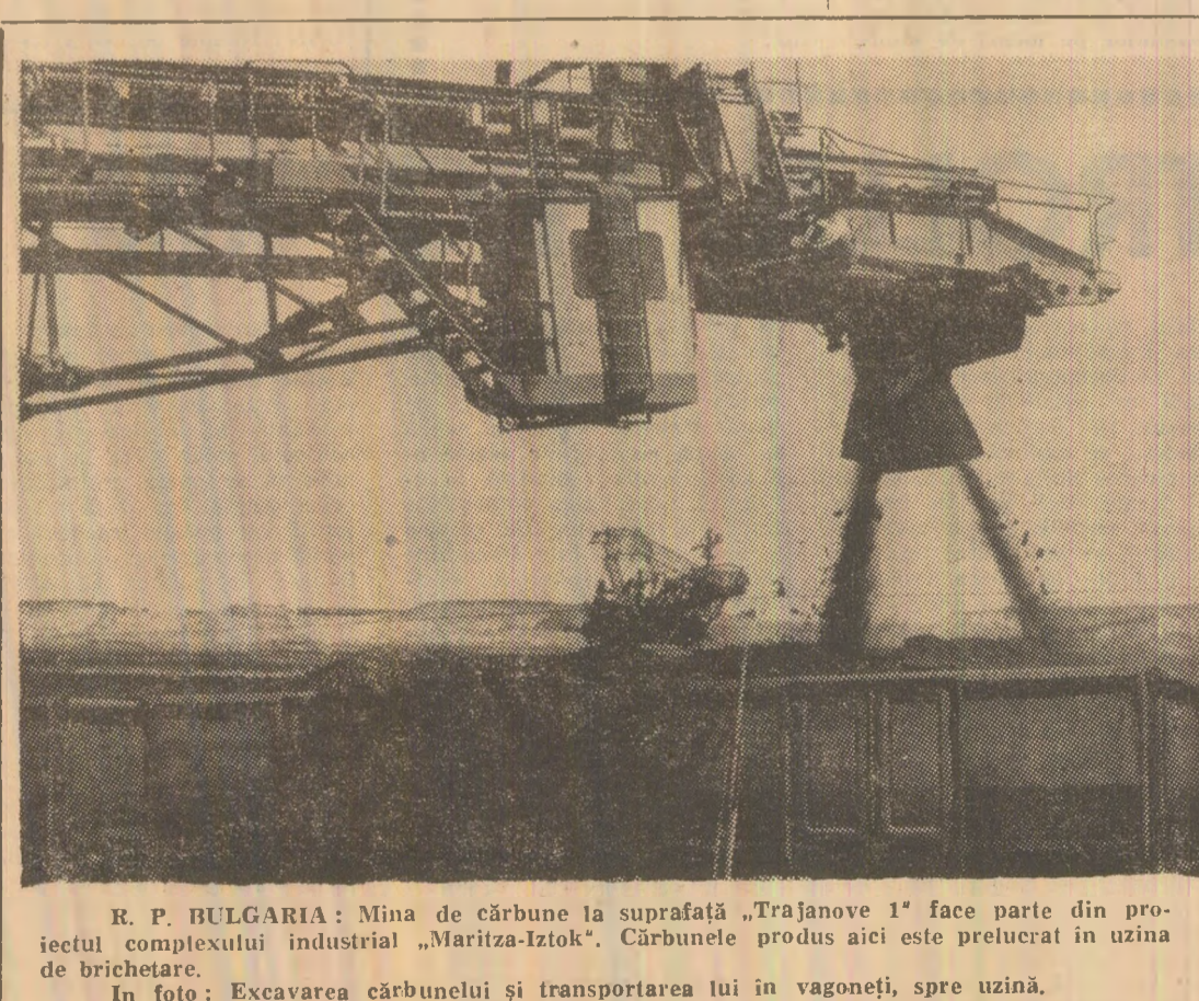
R. P. BULGARIA: Mina de cărbune la suprafață „Trajanove 1” face parte din proiectul complexului industrial „Maritza-Iztok”. Cărbunul produs aici este prelucrat în uzina de brichetare. În foto: Excavarea cărbunului și transportarea lui în vagoane, spre uzină.
