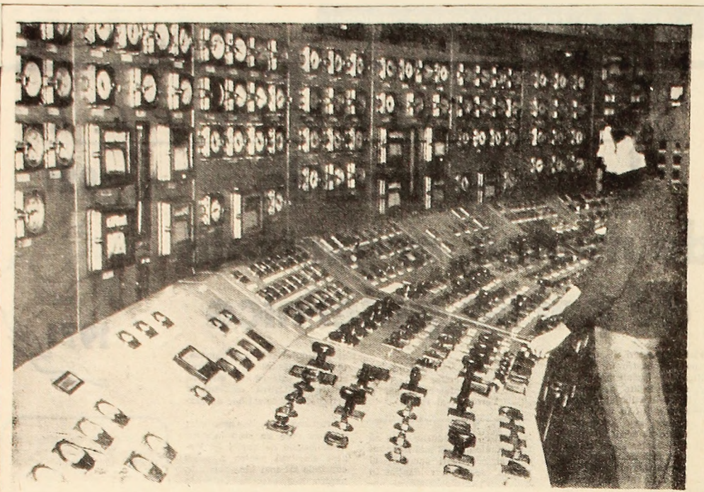
Tehnica modernă, ce permite dirijarea de la distanță a celor mai complexe procese tehnologice, este folosită și la termocentrala Paroșeni. Imaginea fotografică de mai sus înfățișează un astfel de aspect din sala de comandă termică. Foto: N. GHENA
