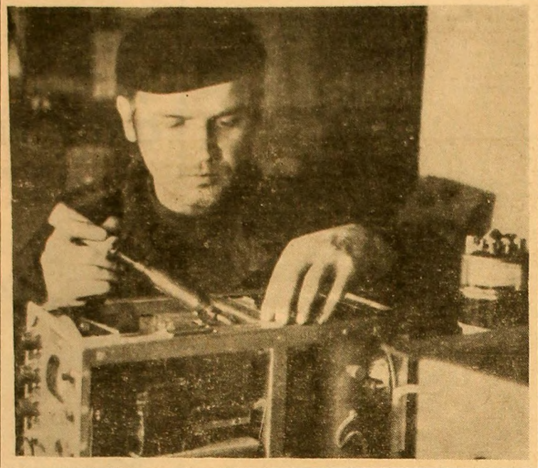
U.U.M. Petroșani: Electronicul Ion Hăluș surprins de obiectiv în timpul reparației unui melanometrul electronic.
