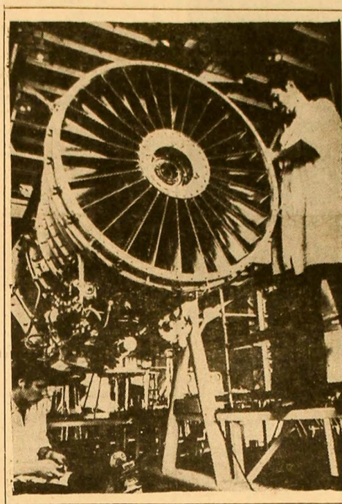
U.R.S.S.: Uzina de motoare de aviație din Perm — una din cele mai mari întreprinderi de acest gen din U.R.S.S. produce motoare cu reacție cu două circuite, care sînt folosite pentru avioanele de pasageri TU-134. Datele calitatilor sale tehnice și de exploatare, noile modele se bucură de apreciere în țară și peste hotare.
