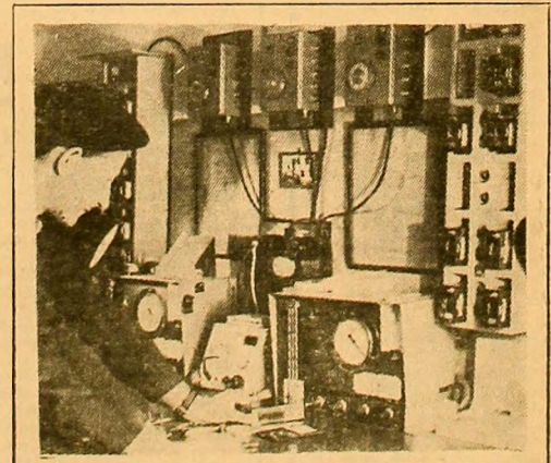
U.U.M. Petroșani. Se execută o verificare a metanometrelor la standul de verificare AUEB. Foto: I. LEONARD
