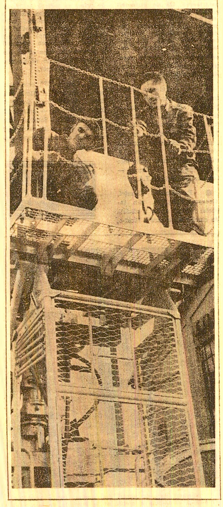
Un nou prototip de utilaj proiectat și executat la U.U.M. Petroșani va lua drumul spre exploatarea minieră din Baia Mare: Dispozitivul de săpare pe verticală denumit „alemacul pneumatic”. În clișeu, mecanicii monteori surprinși în timpul finisării și rodării utilajului reamintit.
