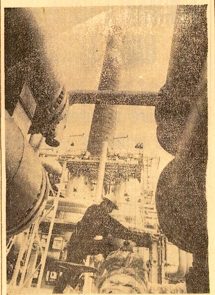
R.S. CEHOSLOVACA. În prezent la uzina petrochimică SLOVNAFT din Bratislava se execută importante lucrări de extindere. În foto: Instalațiile de redistilare din cadrul uzinei petrochimice SLOVNAFT, din Bratislava.
