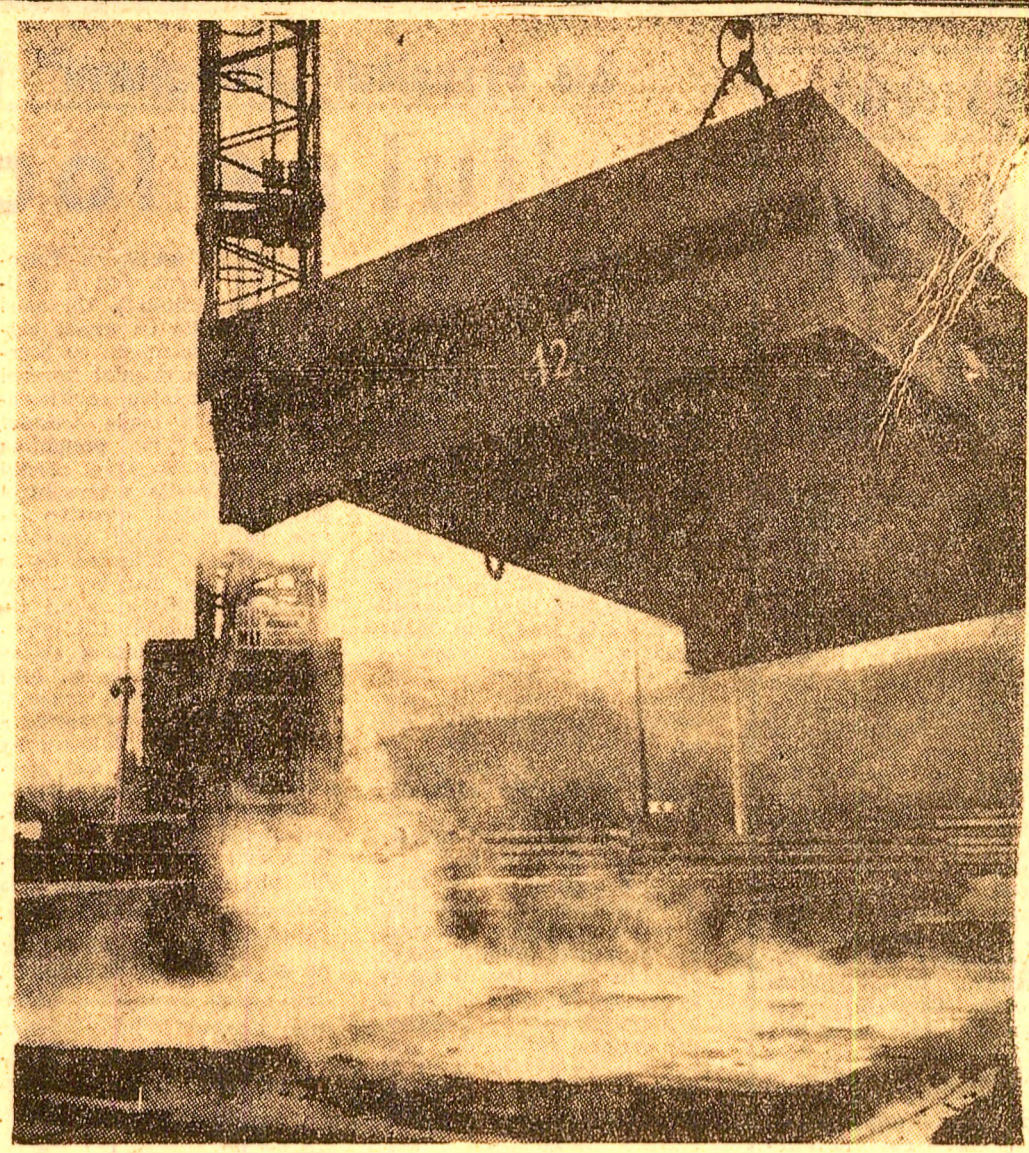
POLIGONUL DE PREFABRICATE LIVEZENI. Acoperirea planșelor de beton cu perne de aburi pentru a fi izolate de frig țace parte din tehnologia de lucru a prefabricatelor. În clișeu, ridicarea pernei de pe „corpul” panoului care încă aburește.
