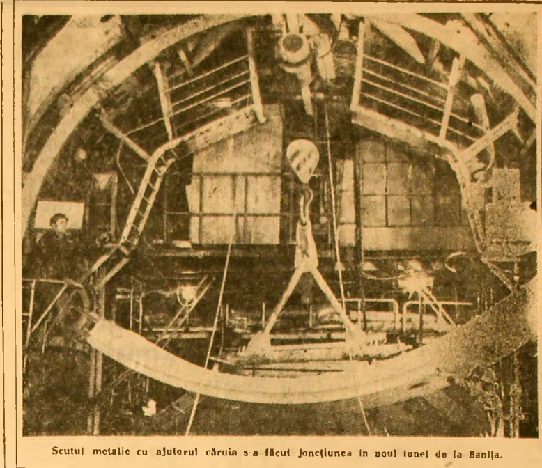
Scutul metalic cu ajutorul căruia s-a făcut joncțiunea în noul lunel de la Banja.
