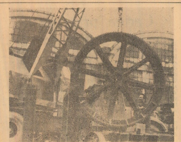
Se montează în incinta U. U. M. Petroșani troliul pentru funicularul de haldare al minei Petrița de către echipa de lăcătuși-montori condusă de Alexandru Pogăceanu.
