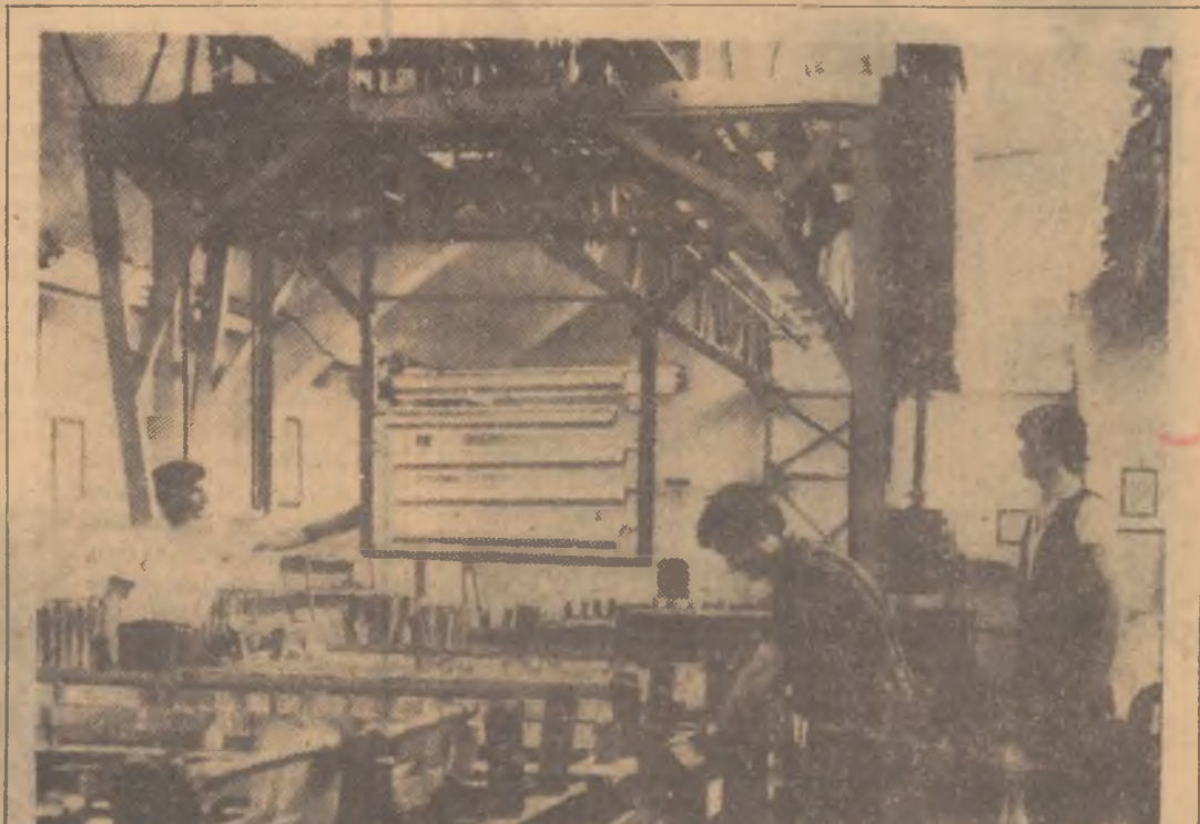
În hala de galvanizare și cadmiere a E.S.H. Vulcan — una din secțiile în care domnește ordinea și disciplina i-am înregistrat pe Ion Zburlea, Nicolae Ghiocșa și Dumitru Turcu în timpul operației de galvanizare a telescoapelor, pentru stilpii hidroaici.
