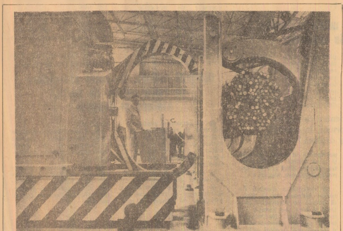
Combinatul de construcții de mașini grele din Magdeburg, R.D.G. În FOTO: Instalația de împachetat bare de oțel, echipată cu o mașină de strîns.
