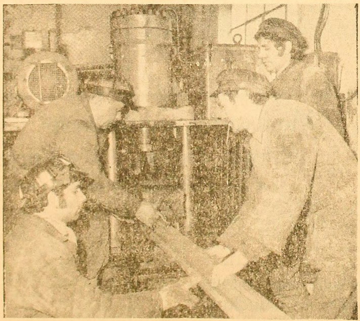
E. M. Lonea La presa hidraulică pentru confecționarea armăturilor T. II. am surprins echipa condusă de Emil Protopopescu în timpul execuției unor armături circulare de susținere în galerii. foto: Ion LICIU
