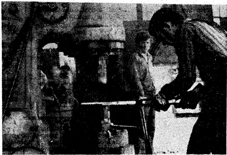
Atelierul electromecanic al I. M. Uricani. Comunistul Ion Iacob, șeful secției forță execută eclise pentru calea ferată din subteran.
