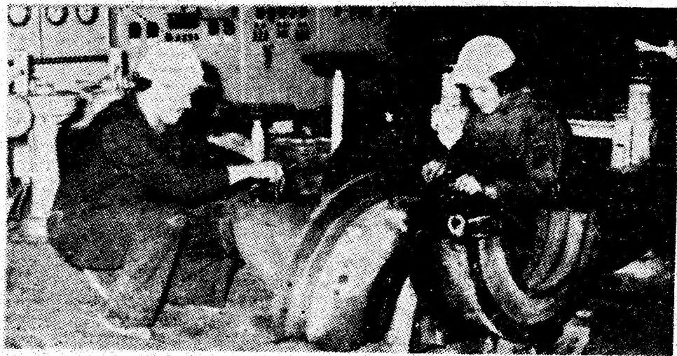
Lăcătușii Constantin Brinzăianu și Vasile Sfarț de la U.E. Paroșeni se ajută reciproc la modificarea instalației uneia din turbinele generatoare, care vor livra în viitorul apropiat, pe lângă energie electrică și energie termică.
