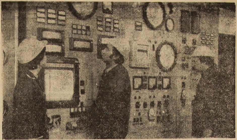
Seful de echipă Titu Birăn și muncitorii PRAM-ști Dorina Mureșan și Emil Pop verifică funcționarea corectă a aparatelor de măsură și control de la pupitrul de comandă a grupului nr. 2 de 50 MW de la U.E. Paroșeni.
