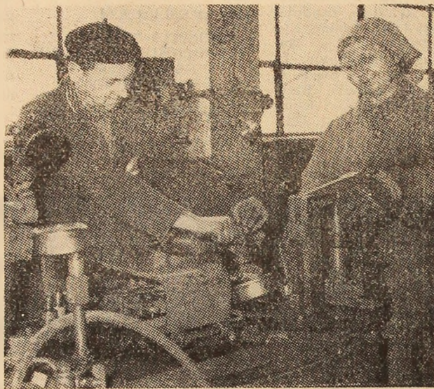
Șeful de echipă lăcătuș Dănilă Matei și muncitoarea Olga Oraveț verifică un set de ventilatoare de siguranță la standul de încărcare cu azot, dispozitiv conceput și realizat la atelierul mecanic al minei Lupeni. Foto: Ștefan NEMECSEK
