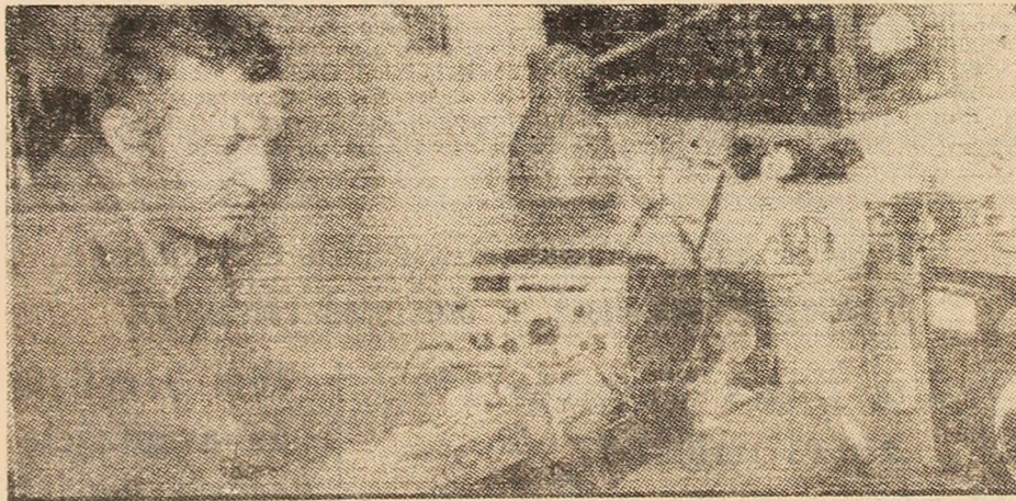
Aspect de muncă din cadrul Atelierului de telegizumetrie de la I.M. Aninoasa. În imagine electronistul Dumitru Vilciu verifică un set de capete de detecție ale stației telegizumetrice. Foto: Ion BALOI
