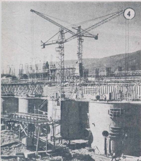
3. De jos, din apropierea tunelului ieșire, țîșnește în sus, prin stielul masiv al muntelui, pînă ce ochiul vede cerul, castelul de echilibru înalt de 100 m
