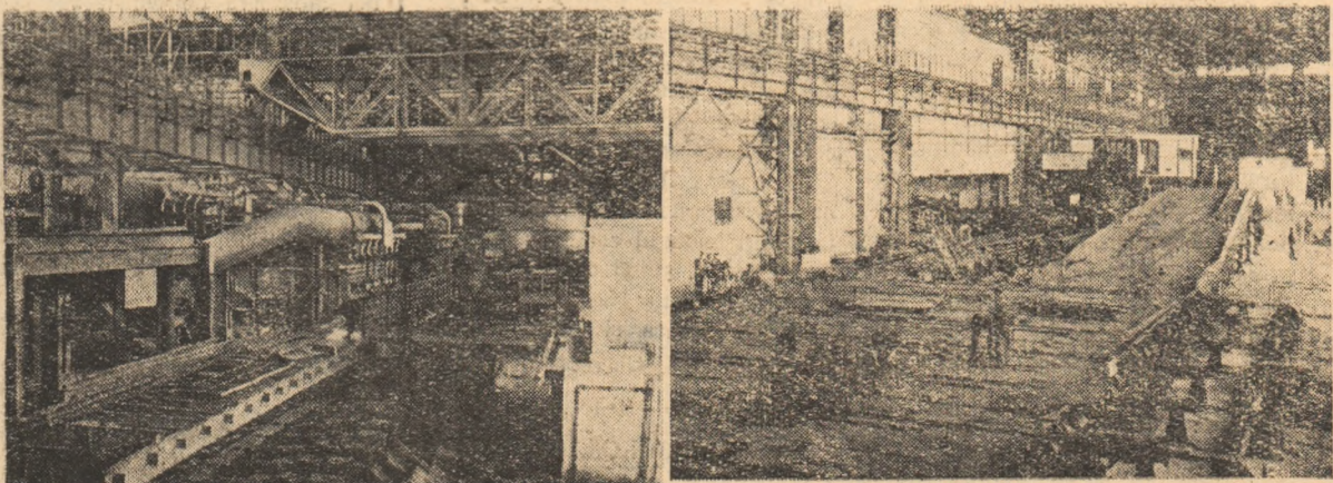
De curînd a intrat în funcțiune laminorul de 850 mm. de la Hunedoara. ÎN FOTO: cuptoarele cu propulsie și linia de laminare.
