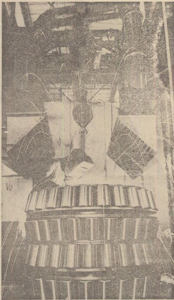
Un rulment de 4.000 de kilograme? Iată-l pregătit pentru asamblare în secția de sudură a Uzinei de rulmenți nr. 1 din Moscova. În această uzină, cele mai multe procese de producție sînt mecanizate.
