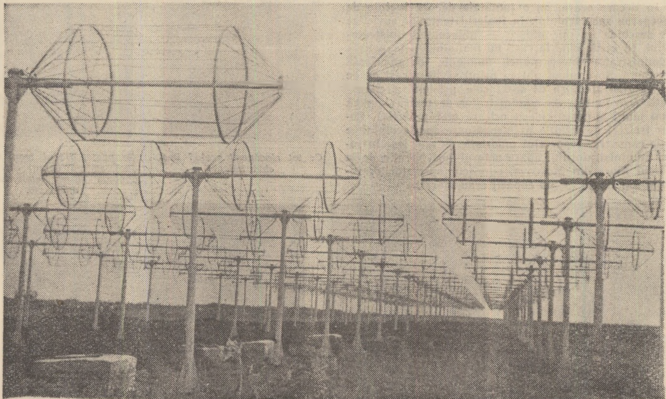
Puternicul radiotelescop al Academiei de Științe a R. S. S. Ucrainene interceptează semnale din constelația Lebede situat la o depărtare de 300.000.000 ani lumină.
