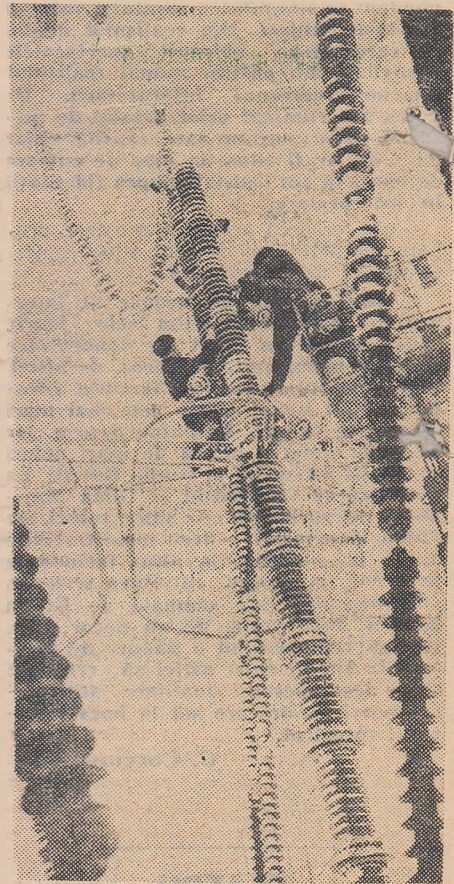
Înterupătorul de înaltă tensiune, o verigă importantă în lanțul transmiterii energiei electrice.
