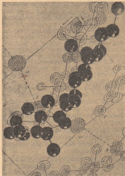
Ultimul pas : modelul moleculei construit peste „curbele de nivel” care desemnează poziția atomilor
